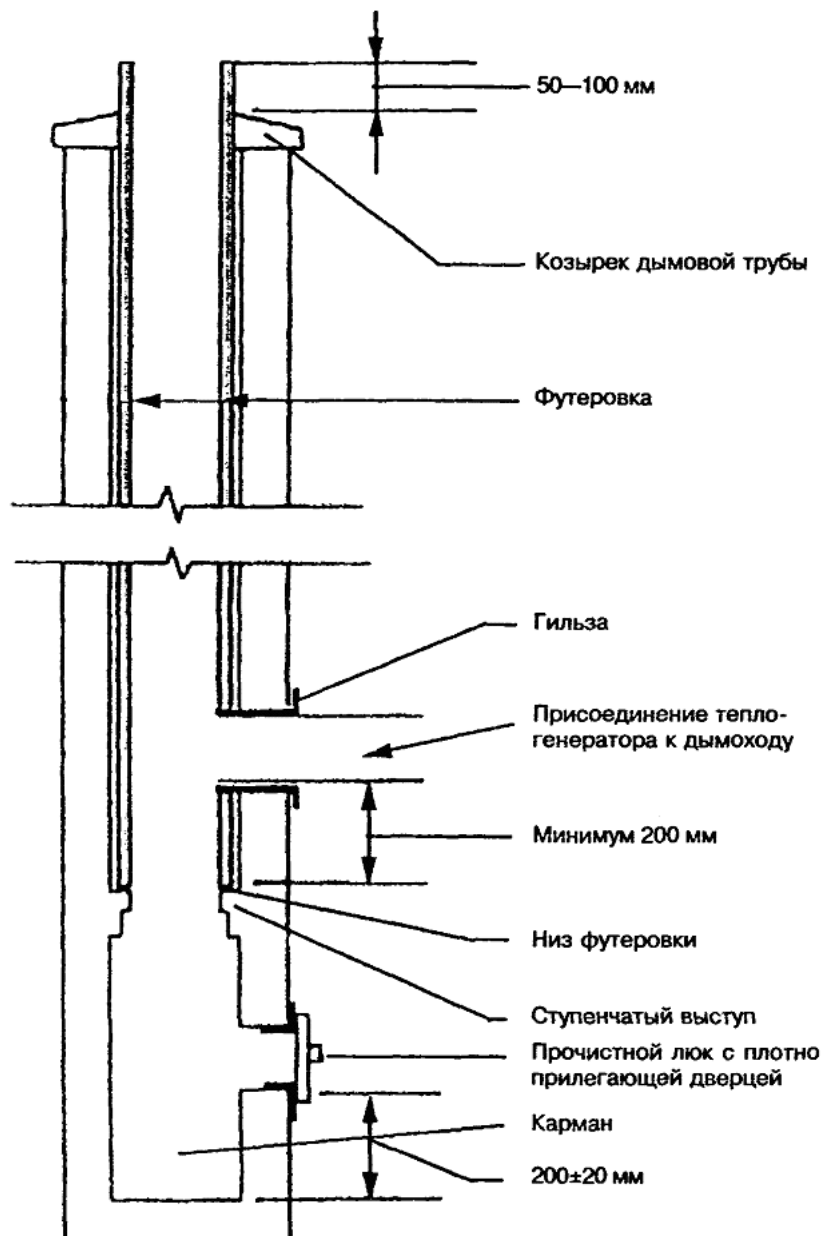
Рисунок 7.5 - Футеровка камина
