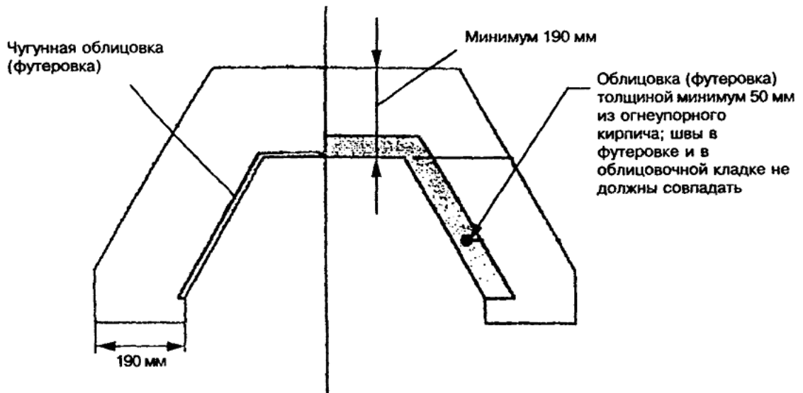
Рисунок 7.5 - Футеровка камина
