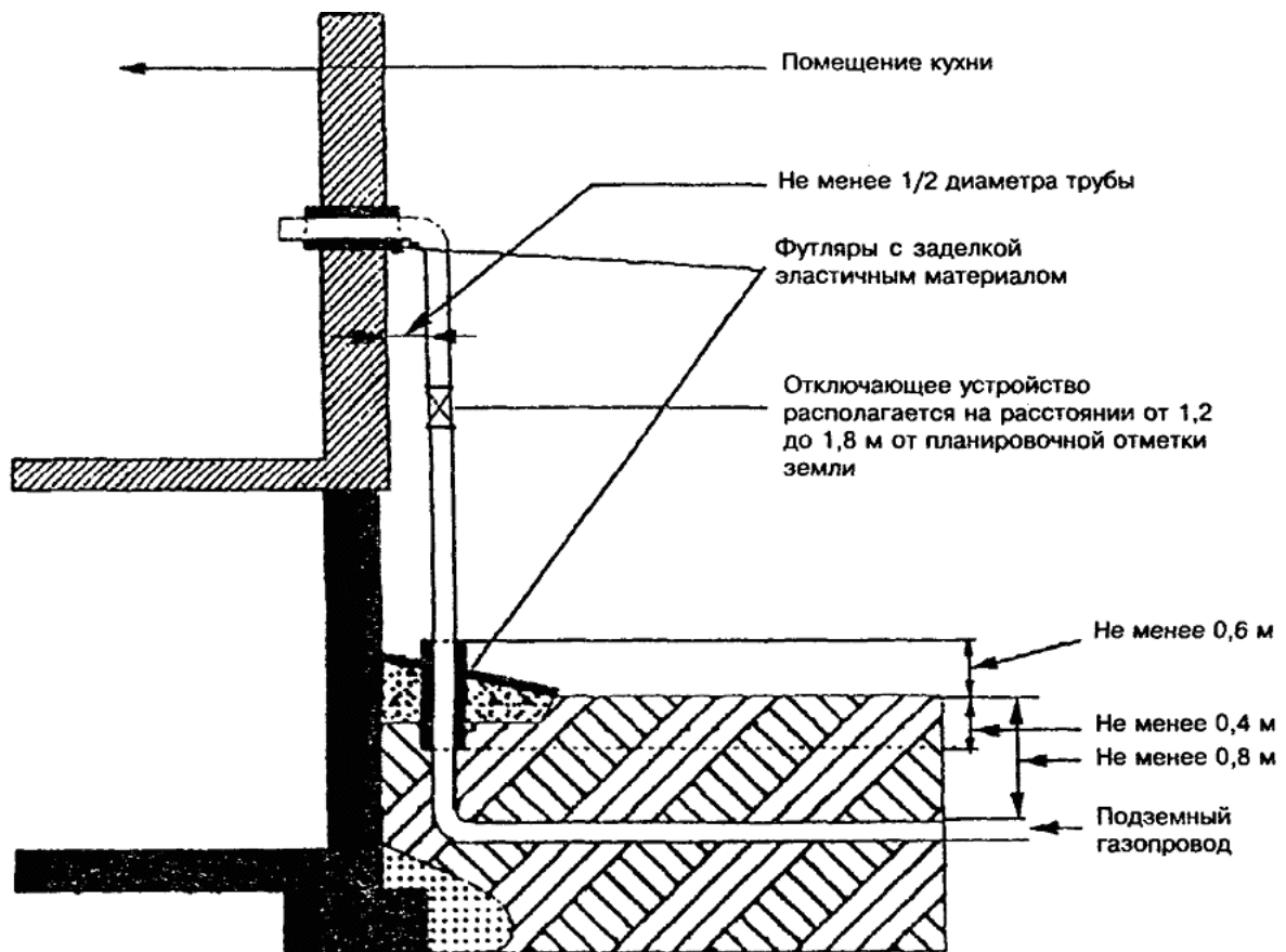
Рисунок 9.1 - Газовый ввод
